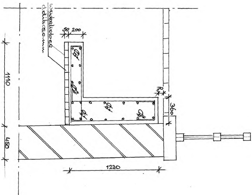
Doorsnede B Schaal 1:20
